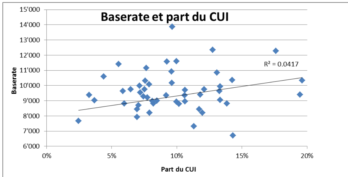
Graphique 2 : rapport entre la part des coûts d'utilisation des immobilisations (CUI) et le baserate (base de référence : coûts d'exploitation nets 1, coûts d'utilisation des immobilisations inclus)
